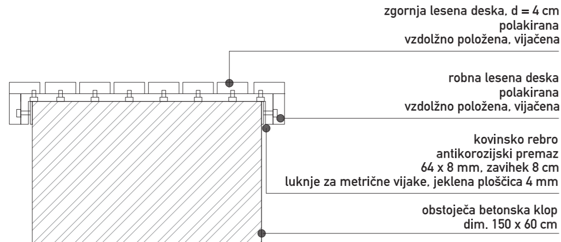
PREČNI PREREZ
