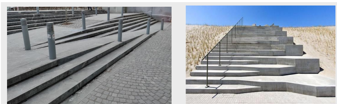
Sliki 9: 1 (neustrezno) Stopnišče z integrirano klančino je vključujoče le na prvi pogled, sicer pa je za večino uporabnikov s funkcionalnimi oviranostmi neuporabno, saj so klančine neustrezno opremljene, robovi klančin so nezaščiteni, za slabovidne pa je zelo otežena zaznava robov stopnic. 2 (ustrezno) Stopnišče z izraženo glavno smerjo hoje, ki jo poudarja oprijemalo. Pot po kompleksnih stopniščih je tako lažja (opomba: manjkajo kontrastni robovi stopnic) (vir: https://pin.it/dpoptvU ).
