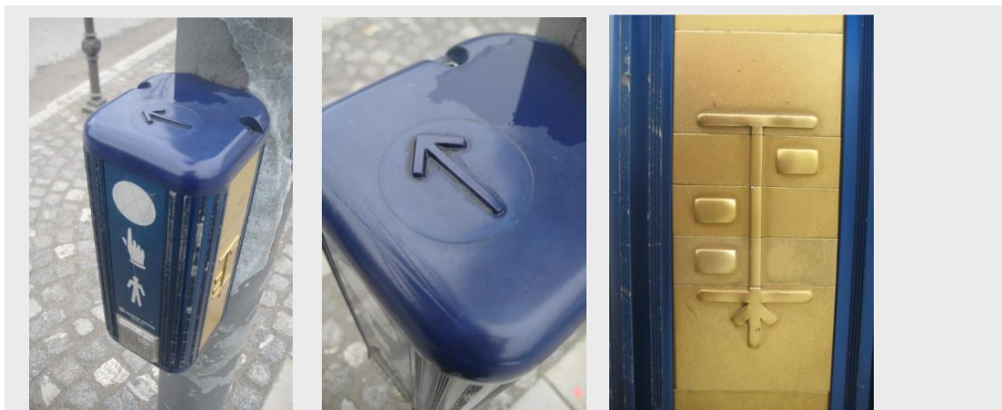
Slike 11 (ustrezno): 1: Zvočni semafor. 2: Reliefna puščica na vrhu škatlice semaforja pešcu z okvaro vida sporoča smer v kateri lahko varno prečka cesto. 3: Na navpični stranici škatlice semaforja lahko pešec z okvaro vida otipa postavitev prometnih pasov in dobi občutek o velikosti ceste, ki jo namerava prečkati.
