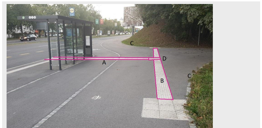
Slika 23 (ustrezno): Primer pripenjanja taktilne oznake vstopnega mesta na vodilno linijo. Oznake vstopnega mesta (A) ni možno pripeti neposredno na rob, zato je izvedena dodatna vodilna linija (B), ki povezuje dva vodilna robova (C). Oznaka vstopnega mesta (A) se na vodilno linijo pripenja s čepastim poljem (D).
